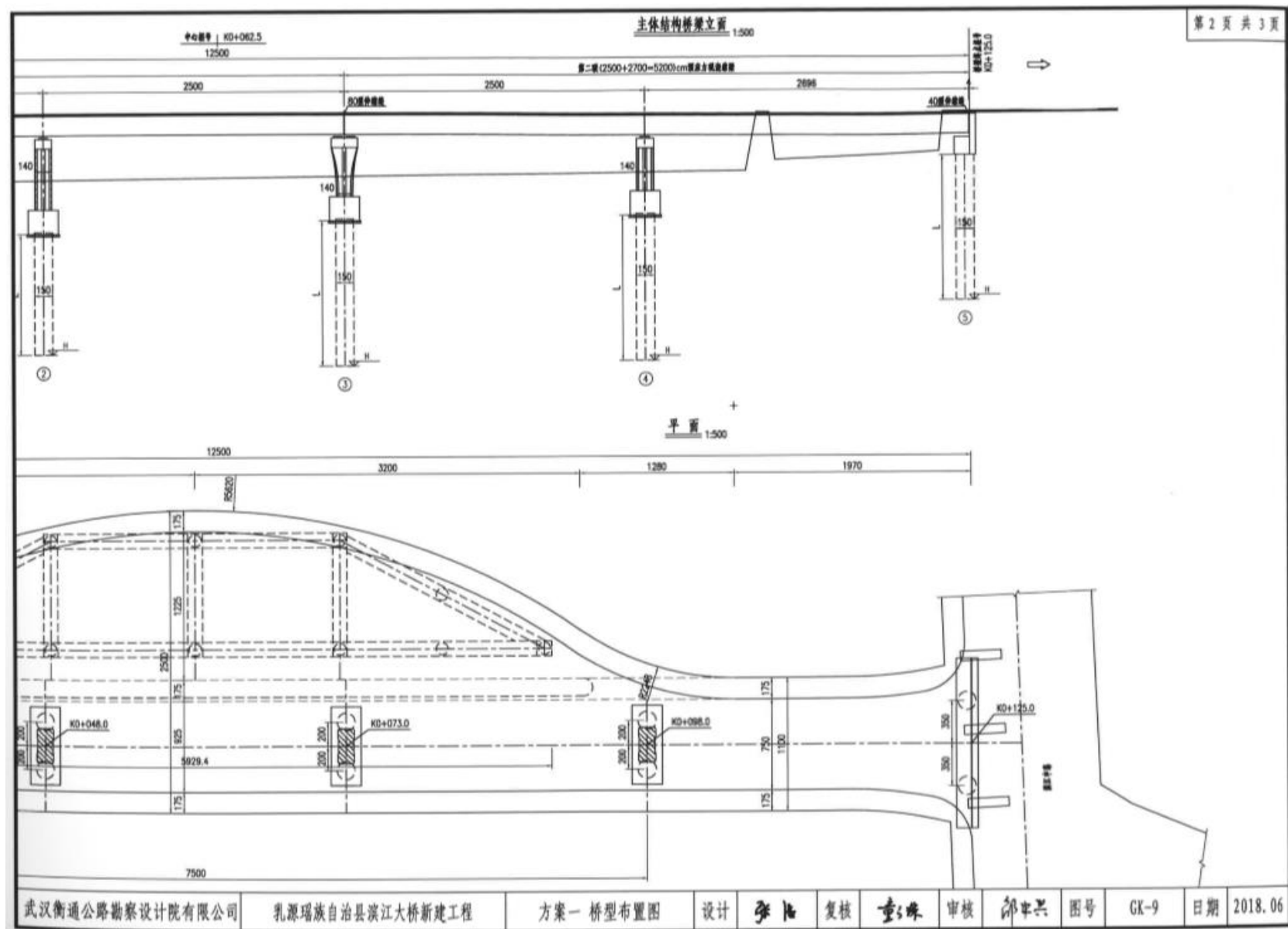
图 6 桥型布置图 (二)
